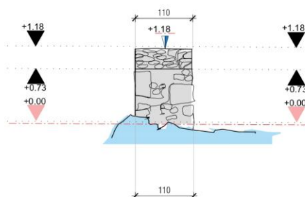
PRERJA B-B PAS RESTAURIMIT SHKALLA 1:70
