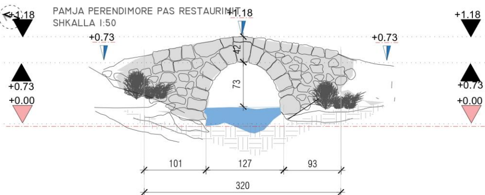
PAMJA LINDORE PAS RESTAURIMIT SHKALLA 1:50
