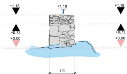
PRERJA A-A PAS RESTAURIMIT SHKALLA 1:70
